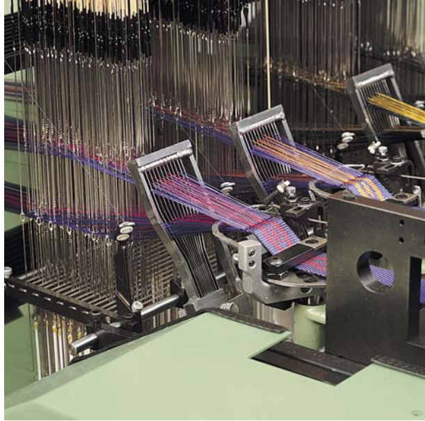
Değişken bant enleri için Y şeklindeki dokuma tarağı dar-geniş-dar
