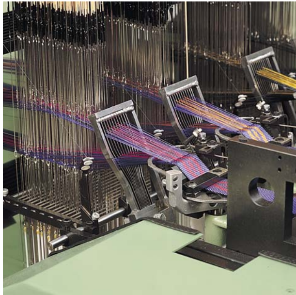
Y-förmiges Webblatt für variable Breite schmal-breit-schmal
