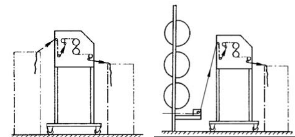
Unidad móvil separada MÜTHERM 2/450 y dispositivo acoplada
