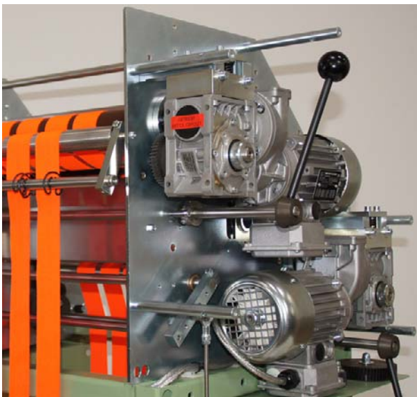
Motores regulados individualmente para los cilindros de entrada y salida
