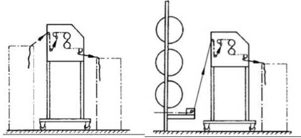
MÜTHERM 2/450: bağımsız, mobil ünite ile birimine bağlı ünite
