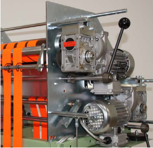
Ayrı motorlarla kumanda edilen giriş ve çıkış silindirleri
